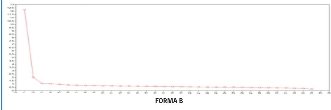
Figura H.5 Scree Plot 4.º básico. Matemática, Forma B
