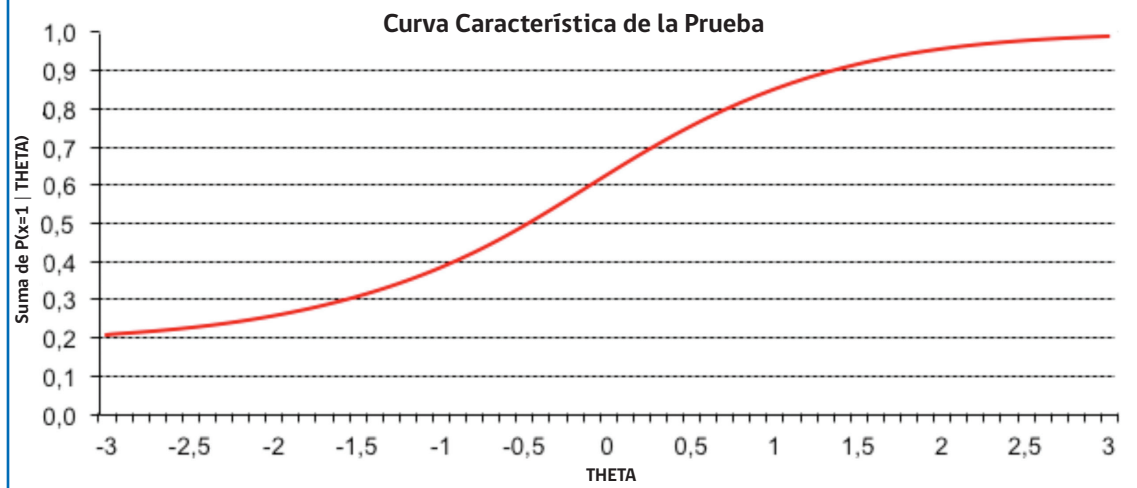
Figura I.3 Curva característica de la prueba, 4.º básico, Lenguaje y Comunicación: Comprensión de Lectura, 2012
