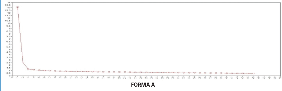
Figura H.12 Scree Plot II medio. Matemática, Forma A
