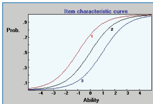
Figura 1.2 Ejemplo de CCI de tres ítems, con dificultad -1,0 ; 0 y 1,0 respectivamente.
