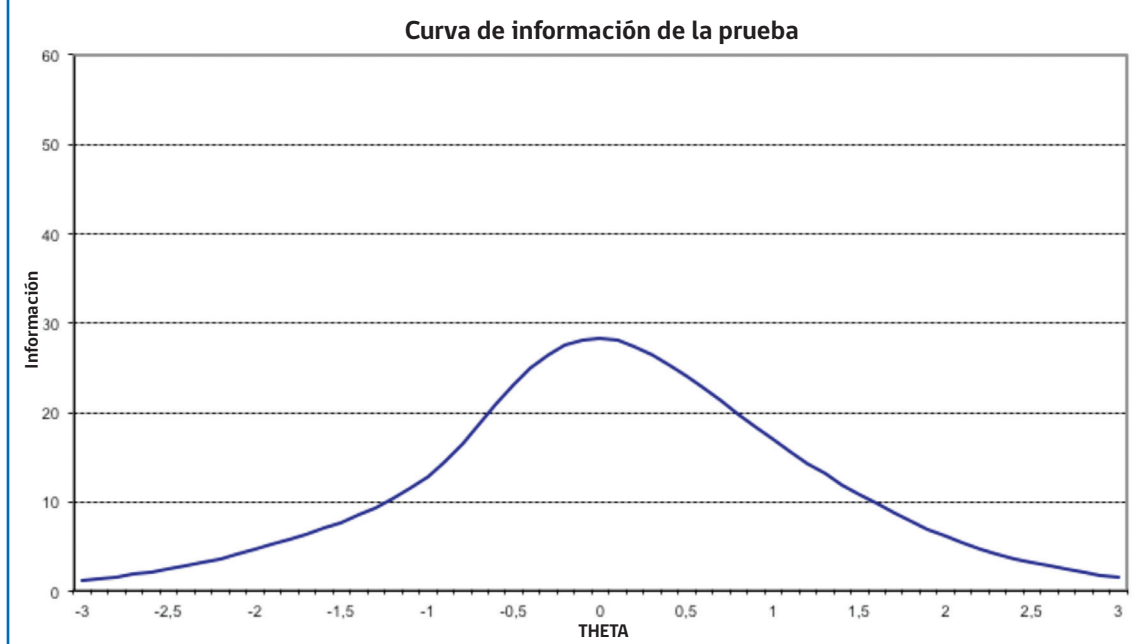
Figura I.4 Curva de información de la prueba, 4º básico, Lenguaje y Comunicación: Comprensión de Lectura, 2012
