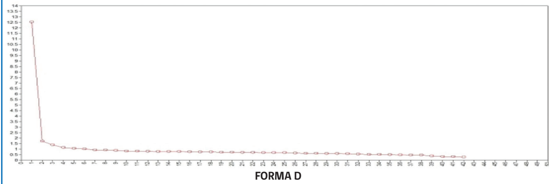
Figura H.15 Scree Plot II medio. Lenguaje y Comunicación: Comprensión de Lectura, Forma D
