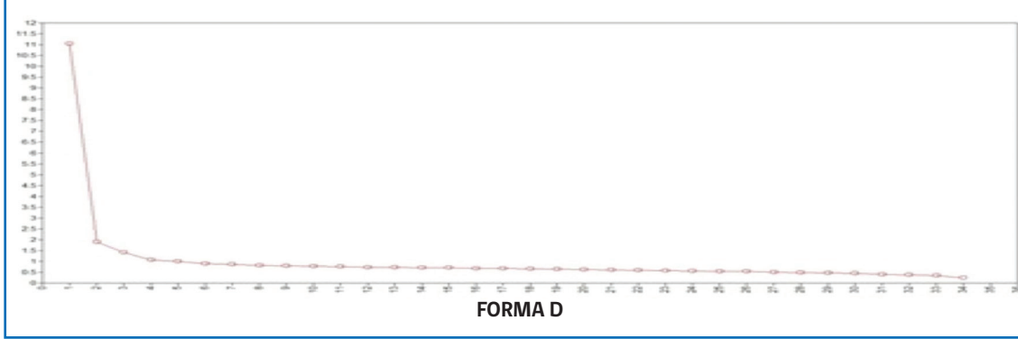
Figura H.7 Scree Plot 4.º básico. Matemática, Forma D
