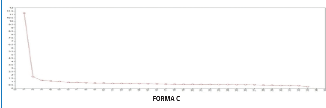
Figura H.6 Scree Plot 4.º básico. Matemática, Forma C
