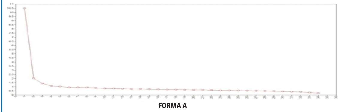
Figura H.4 Scree Plot 4.º básico. Matemática, Forma A
